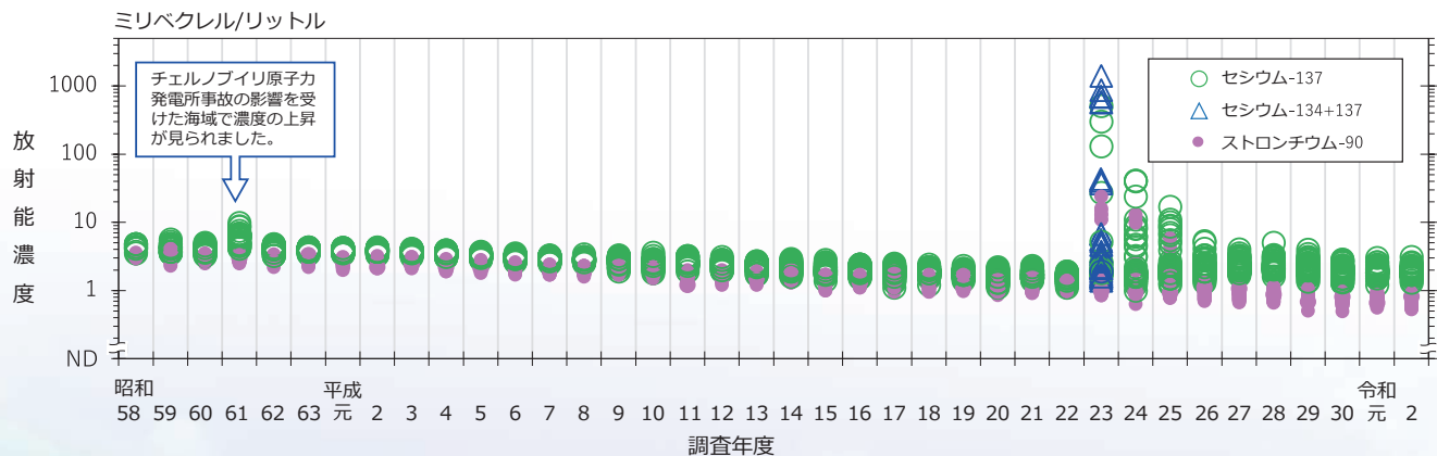
原子力発電所等周辺15海域の海水（表層水）の調査結果
