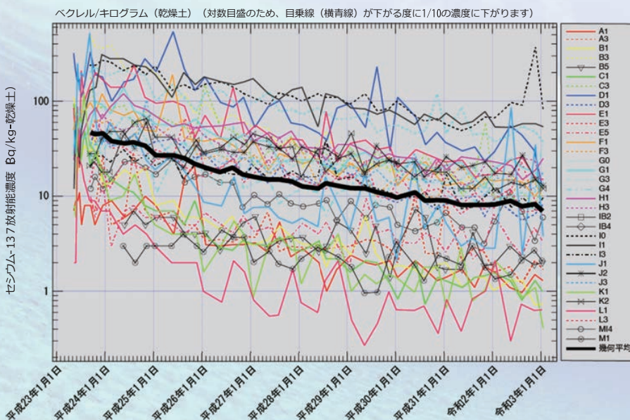
海底土におけるセシウム-137の放射能濃度の変化
