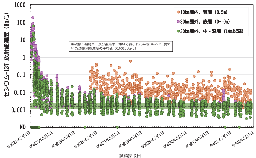
海水中におけるセシウム-137の放射能濃度の変化
