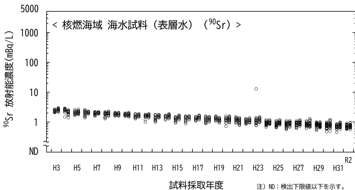
図 I-1-6-66 海水試料の ^{90}\text{Sr} 濃度経年変化（核燃海域・表層水）
