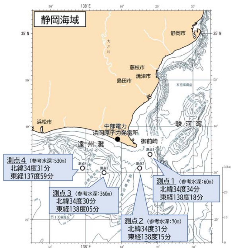
図 I -1-3-6 静岡海域における海底土・海水試料採取測点
