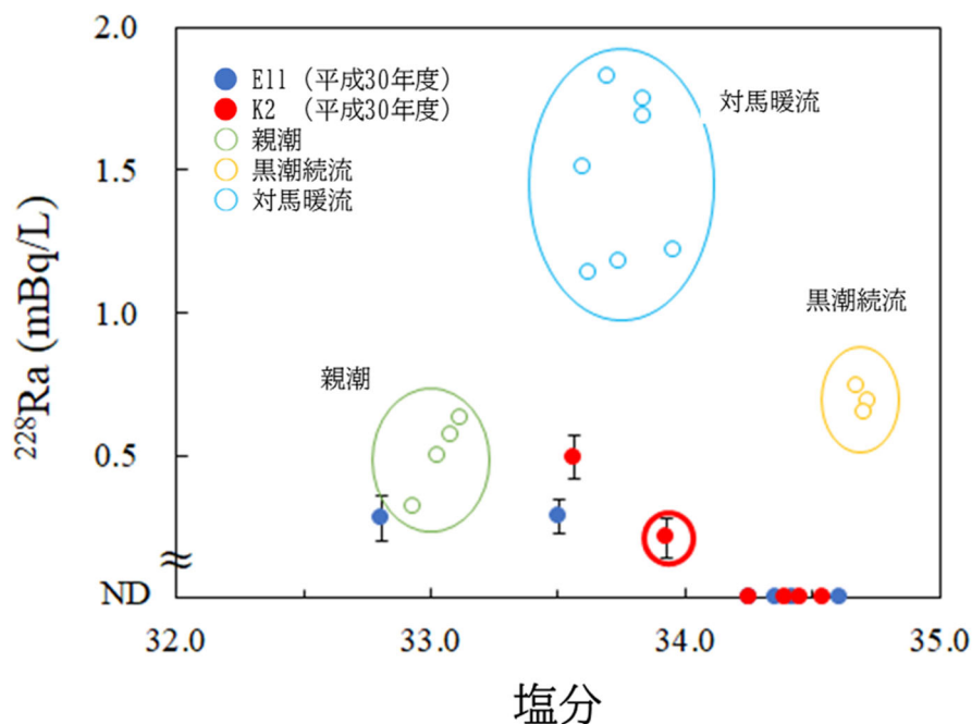
図 I-2-2-3-8 ^{228}\text{Ra} 放射能濃度と塩分の関係。黒潮統流と親潮は Kawakami et al. 21) を、津軽暖流は Inoue et al. 22) を参照した。
