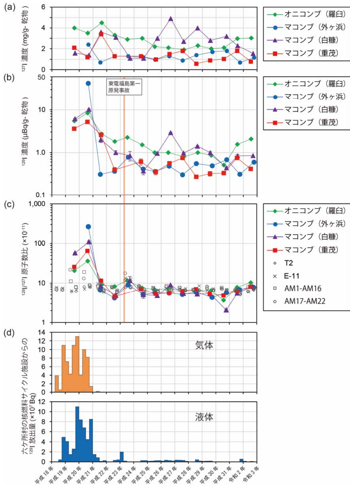
図 I-2-2-2-5 (a)コンブ中の ^{127}\text{I} (安定ヨウ素)濃度、(b)コンブ中の ^{129}\text{I} 濃度、(c)コンブ及び海水中の ^{129}\text{I}/^{127}\text{I} 原子数比、(d)六ヶ所村の核燃料サイクル施設からの ^{129}\text{I} 放出量。AM1-AM16 及び AM17-AM22 における海水中的 ^{129}\text{I}/^{127}\text{I} 原子数比は核燃海域の北部と南部の測点の平均値である。
