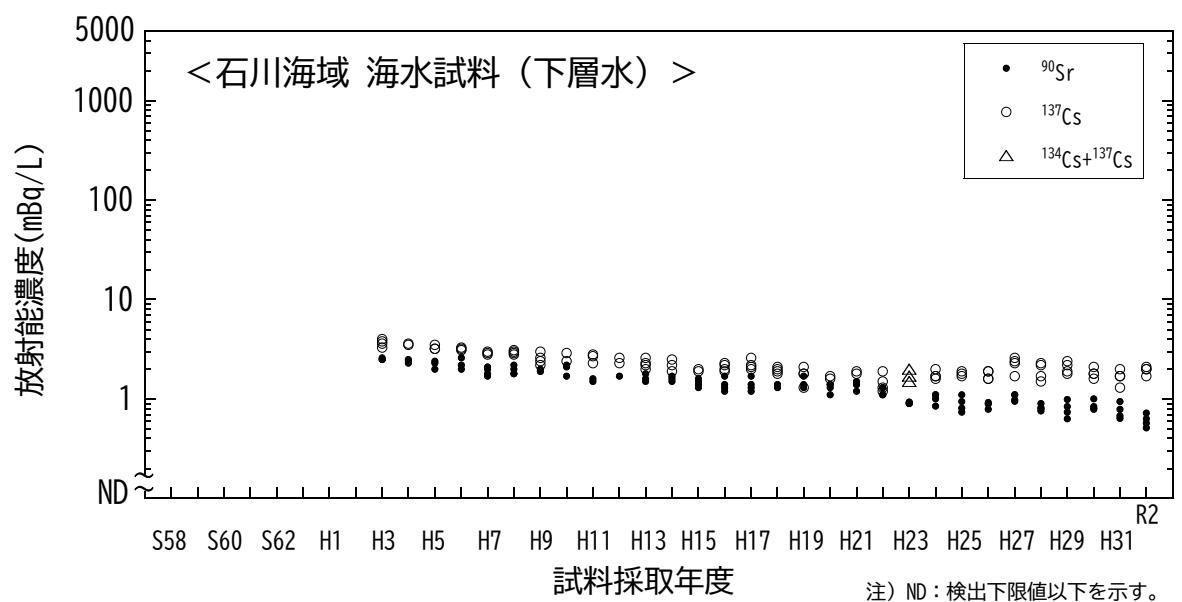
図 I-1-6-47 海水試料の ^{90}\text{Sr} 及び ^{137}\text{Cs} 濃度の経年変化（石川海域・下層水）
