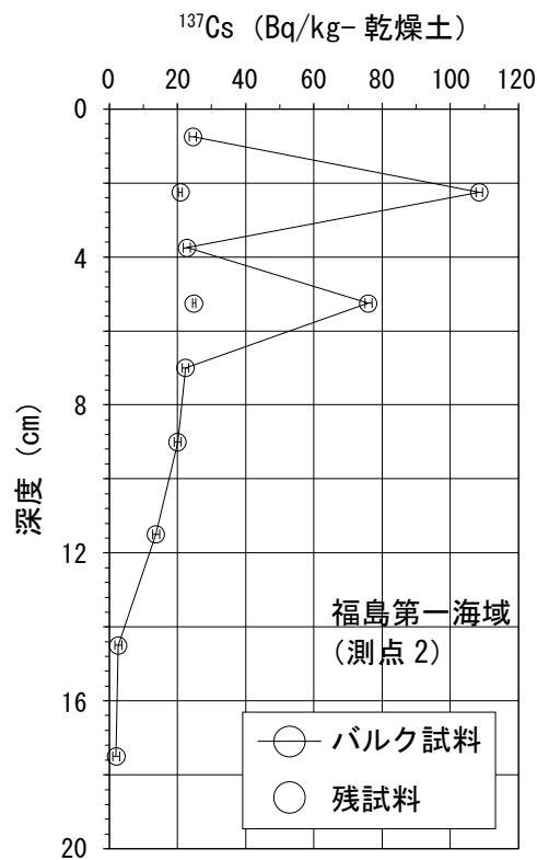
図 I -2-2-3-5 放射性粒子を除く前と後の海底土試料に含まれる ^{137}\text{Cs} 放射能濃度の鉛直分布の変化（誤差は○内に入る）
