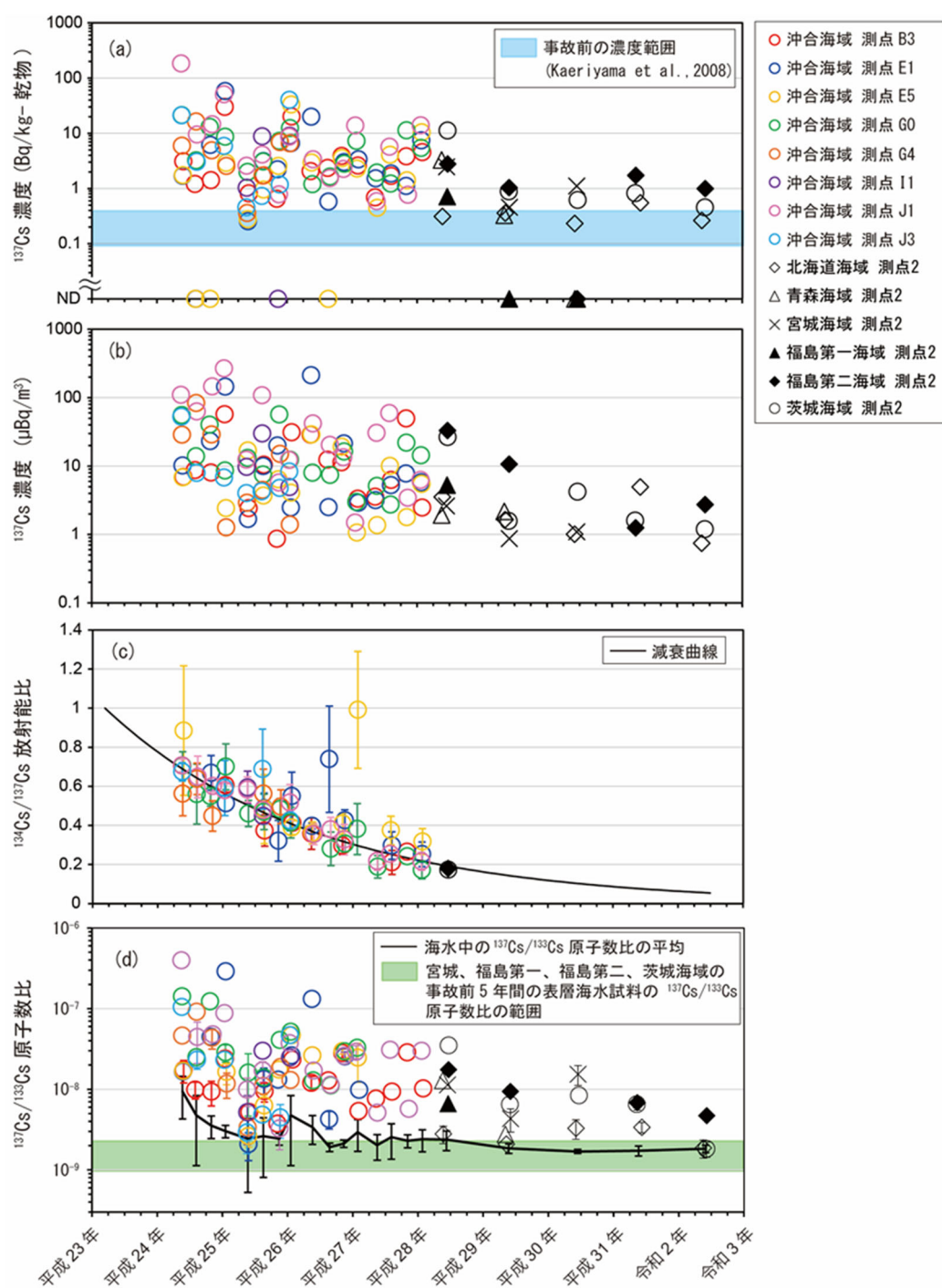
図 I -2-2-3-13 東電福島第一原発事故後の動物プランクトンの放射性セシウムの放射能濃度と ^{137}\text{Cs}/^{133}\text{Cs} 原子数比の時系列変化。(a) 動物プランクトン試料の ^{137}\text{Cs} 放射能濃度(Bq/kg-乾物)、(b) 海水 1 \text{m}^3 当たりの動物プランクトンの ^{137}\text{Cs} 放射能( \mu\text{Bq}/\text{m}^3 )、(c) 動物プランクトン試料の ^{134}\text{Cs}/^{137}\text{Cs} 放射能比、(d) 動物プランクトン試料の ^{137}\text{Cs}/^{133}\text{Cs} 原子数比。ND は測定値が検出下限値以下であることを示す。
