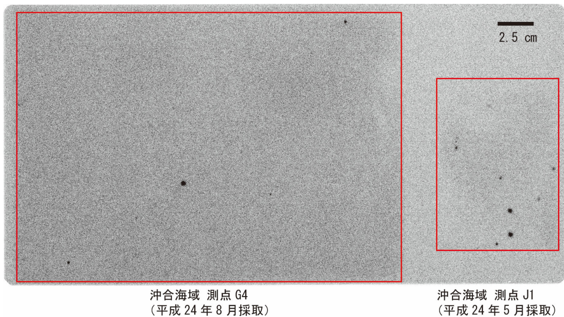
図 I-2-2-3-14 イメージングプレートを用いた計測により得られた動物プランクトン試料のオートラジオグラフ。赤枠の範囲が動物プランクトン試料に該当する。
