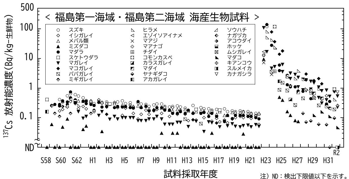
図 I-1-6-4 海産生物試料の ^{137}\text{Cs} 濃度経年変化（福島第一海域・福島第二海域）
