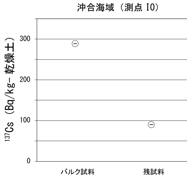
図 I -2-2-3-6 放射性粒子を除く前と後の海底土試料中の ^{137}\text{Cs} 放射能濃度の変化（誤差は○内に入る）
