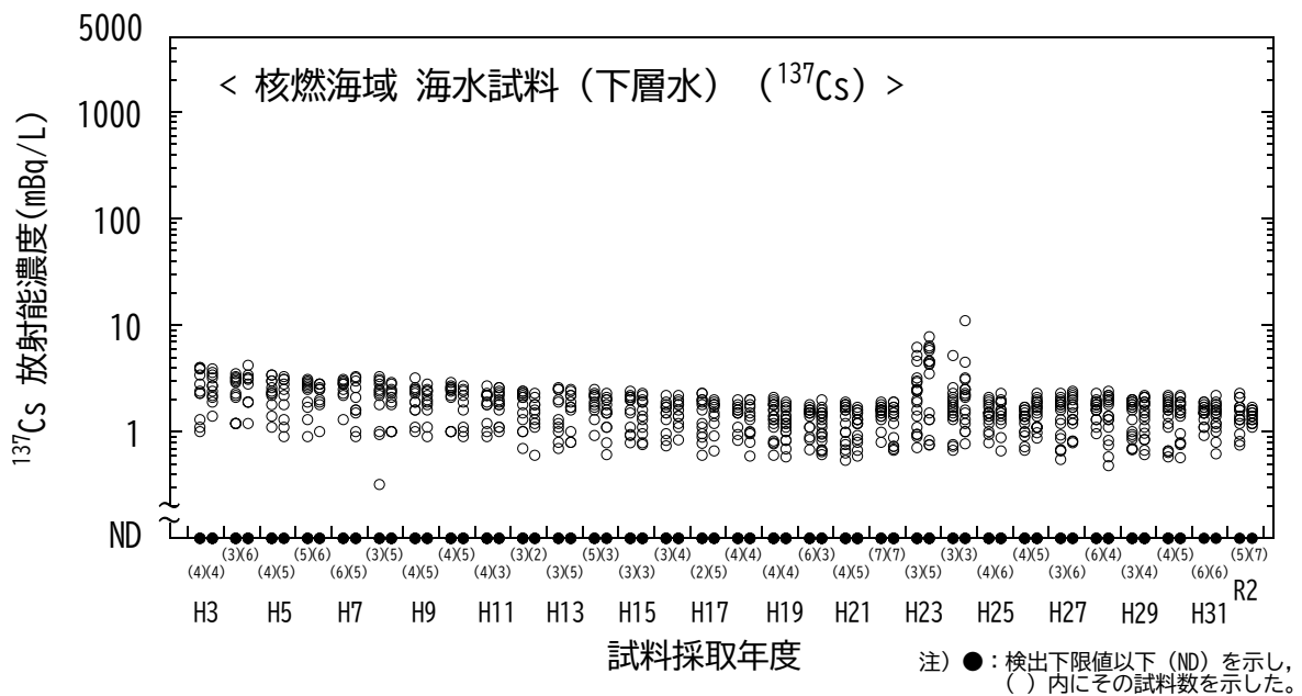
図 I-1-6-69 海水試料の ^{137}\text{Cs} 濃度経年変化（核燃海域・下層水）
