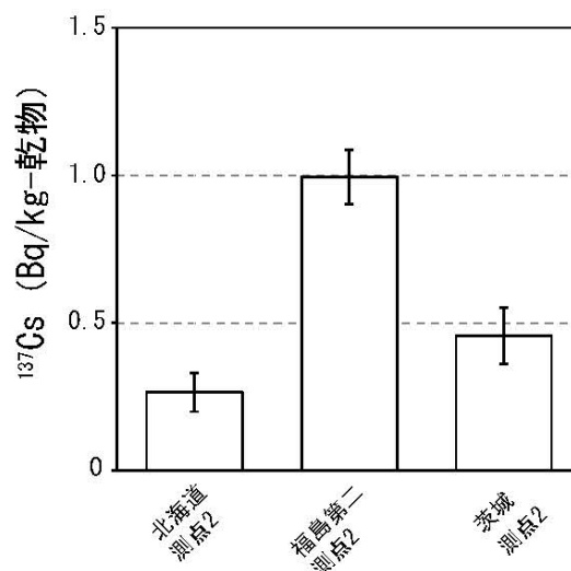
図 I-2-2-3-12 令和 2 年度に各海域の測点で採取した動物プランクトン試料の ^{137}\text{Cs} 放射能濃度（誤差棒は計数誤差を表す）。
