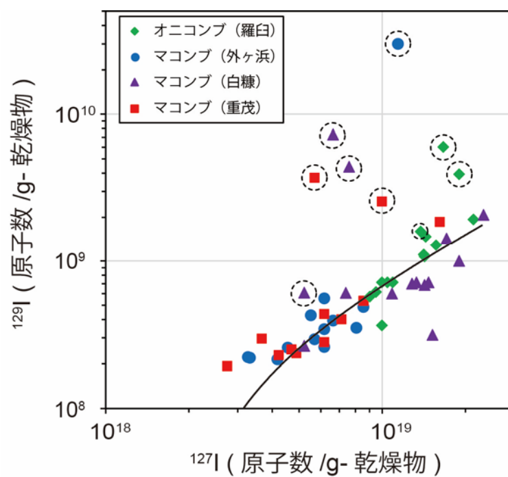
図 I-2-2-2-6 コンプ試料に含まれる ^{127}\text{I} と ^{129}\text{I} の関係。図中の回帰直線は、点線で囲まれたアクティブ試験及び原発事故の影響があるものを除いて計算した。
