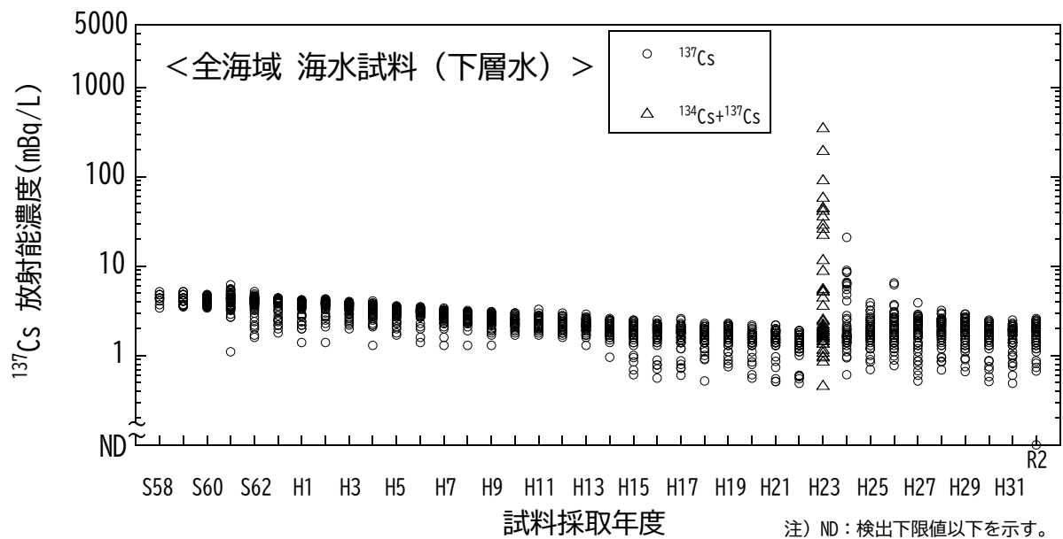
図 I-1-6-31 海水試料の ^{137}\text{Cs} 濃度経年変化（全海域・下層水）
