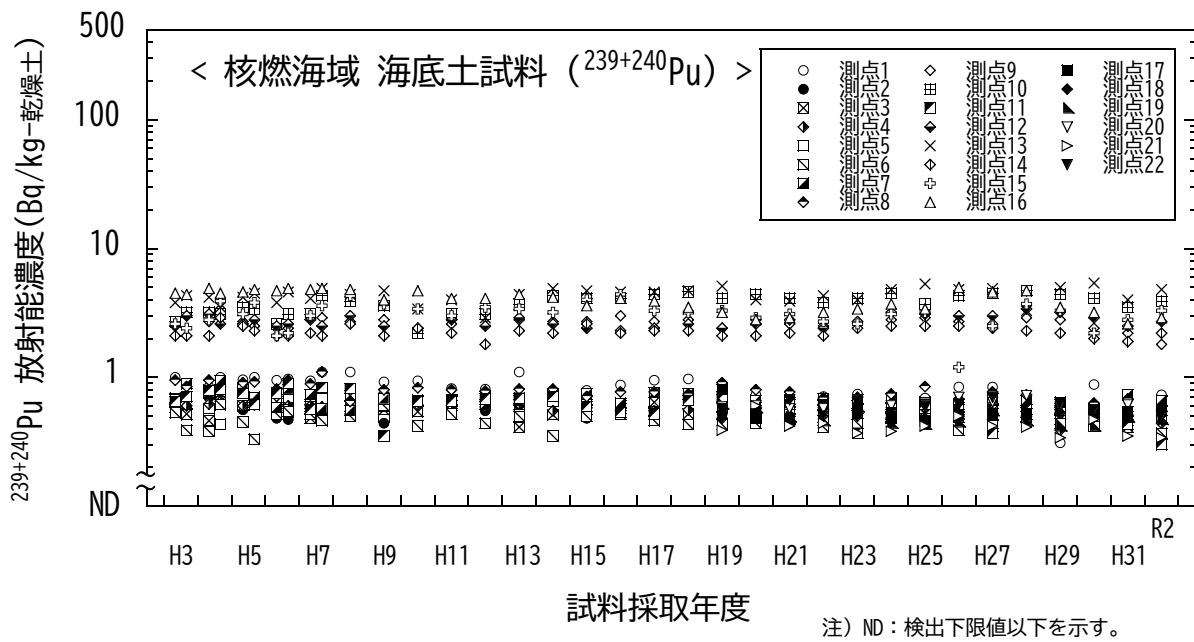
図 I-1-6-63 海底土試料の ^{239+240}\text{Pu} 濃度経年変化 (核燃海域)
