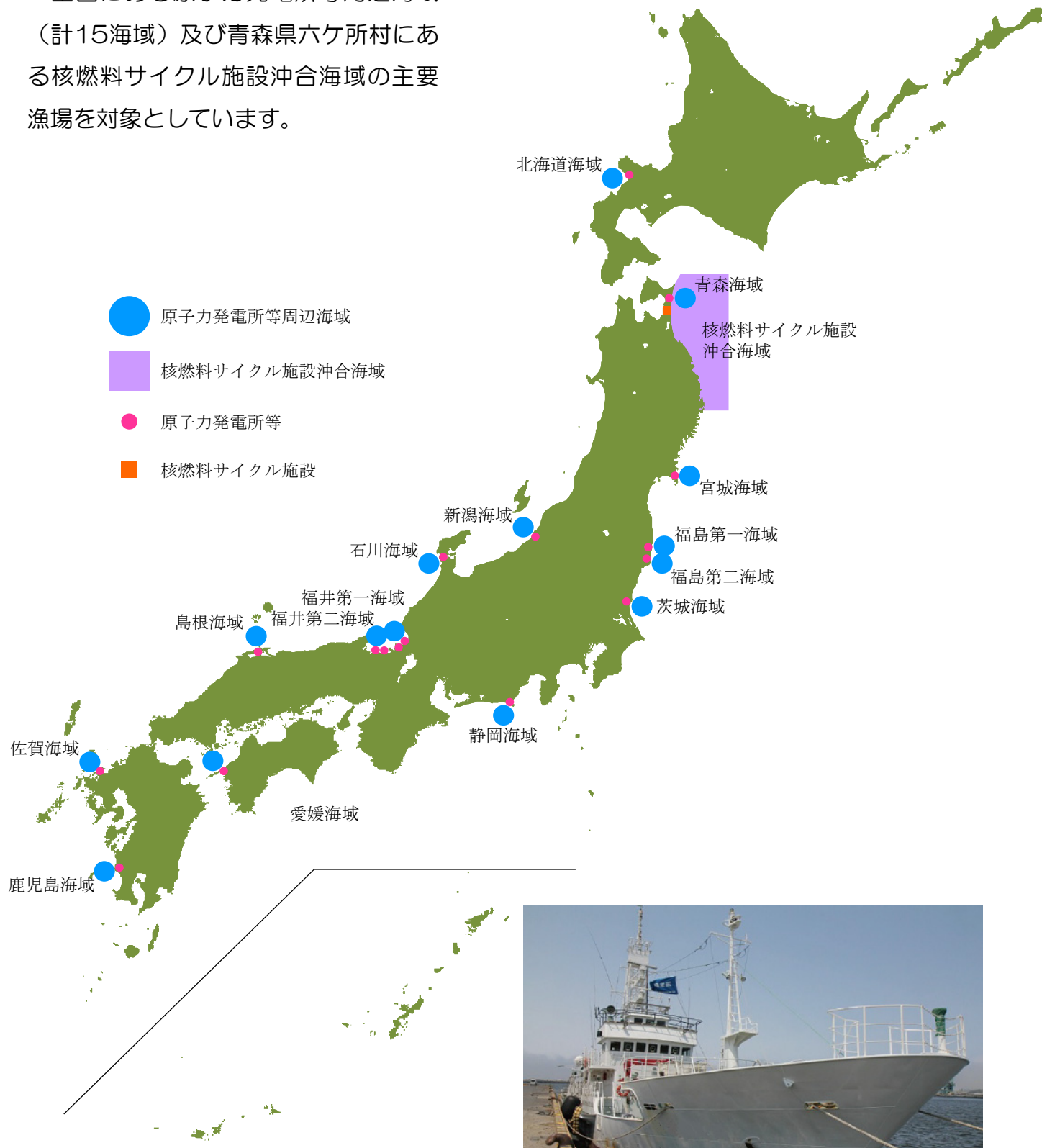
海洋放射能調査に使用した調査船（一例）
