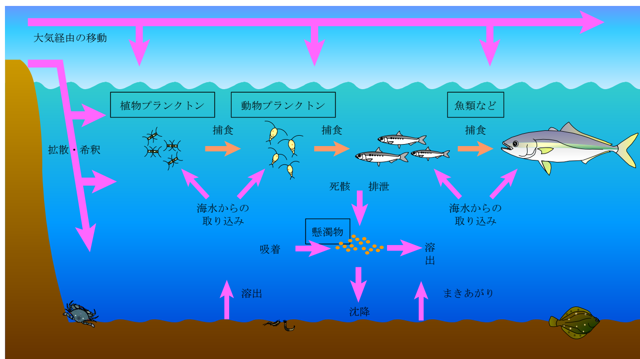
放射性核種の海洋中における動きの概念図
