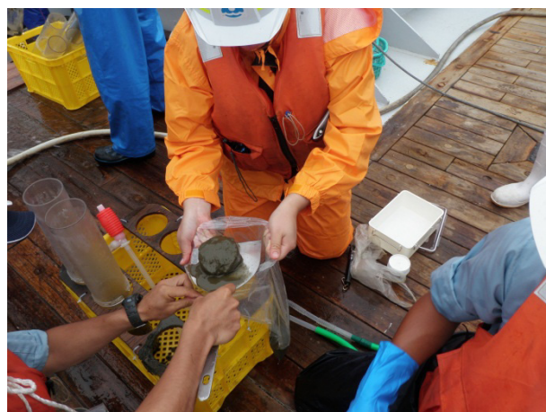
海底土試料の採取作業
