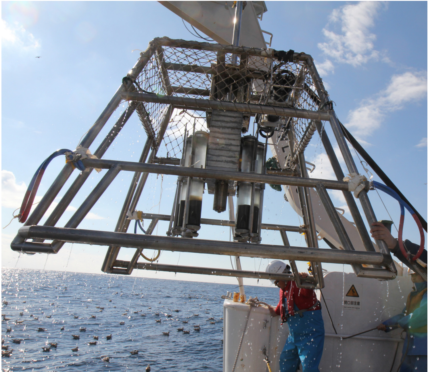
マルチプルコアラーによる海底土の採取
